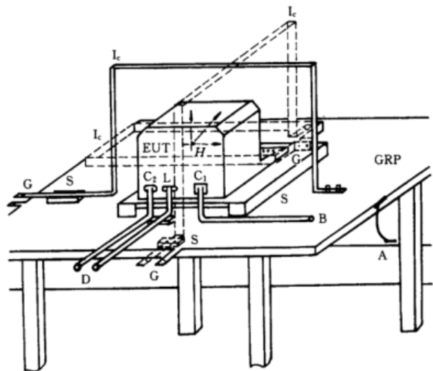
图 4 台式设备的试验布置
